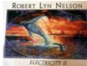
16. Ozeanbild
